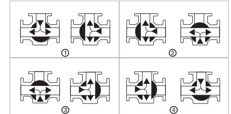
T型三通球阀4种启闭位置
